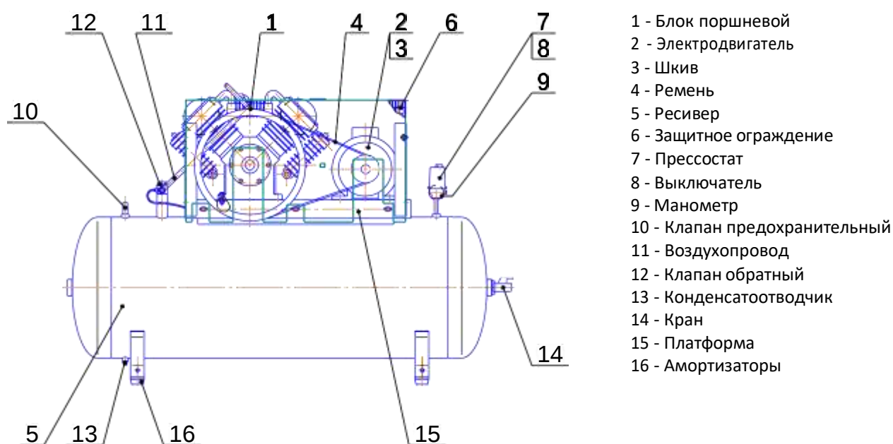
Рисунок 3 - Общий вид компрессоров СБ4/Ф-500.LT100, СБ4/Ф-500.LT100/16-7.5
